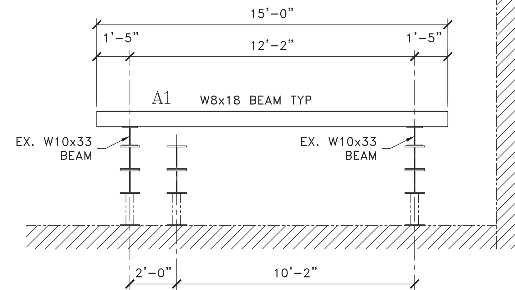
SECTION A-A
